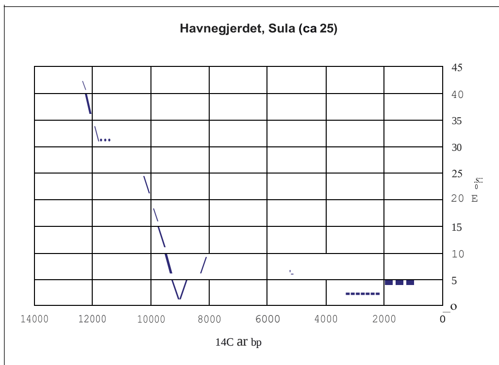
Figur 13: Strandlinjekurve for Havnegjerdet, Sula kommune (kurve 25), etter skjema utarbeidet av David N. Simpson, mars 2001 (jf, Svendsen & Manglerud 1987, Bondevik, Svendsen og Manglerud 1998).
